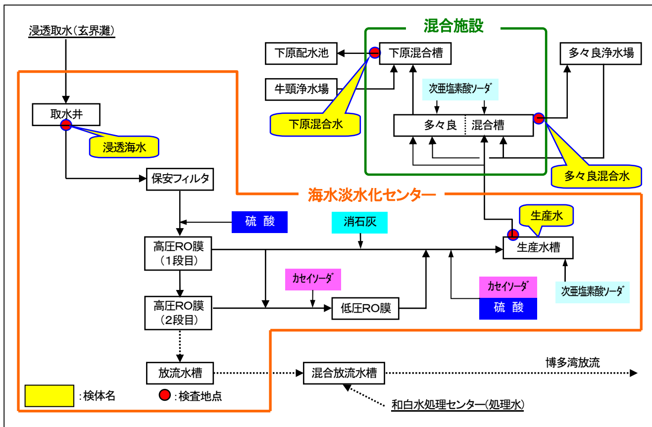
図-4 海水淡水化センター及び混合施設検査地点概要
